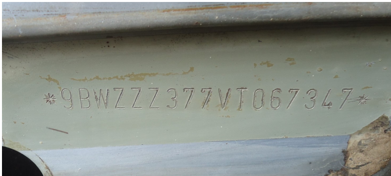
Fotografia nº 02: imagem da numeração de chassi do veículo examinado.
